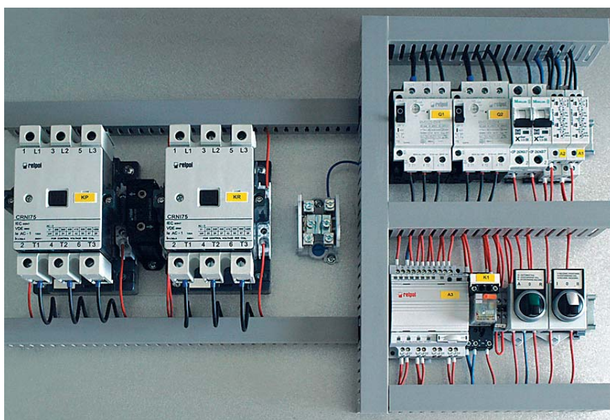
Rys. 3. Moduł po wykonaniu połączeń według dokumentacji jest gotowy do pracy bez dodatkowych czynności programowania czy parametryzacji
